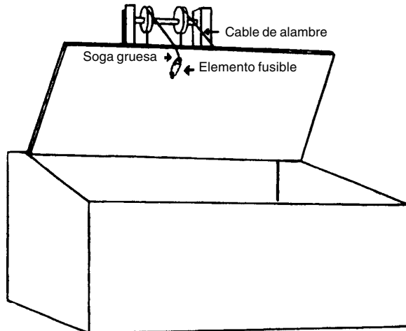
Vista frontal de la tolva de seguridad para materiales de embalaje. Se puede fabricar la tolva de metal o de madera revestida con metal.
